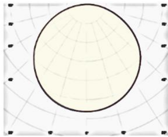
Диаграмма интенсивности светового потока
