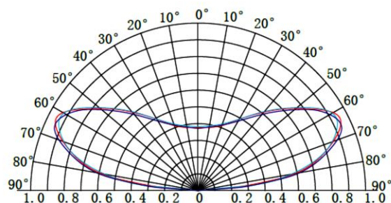
Диаграмма интенсивности свет. потока
