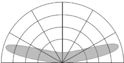
Диаграмма интенсивности светового потока
